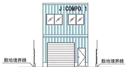
前面立面図
