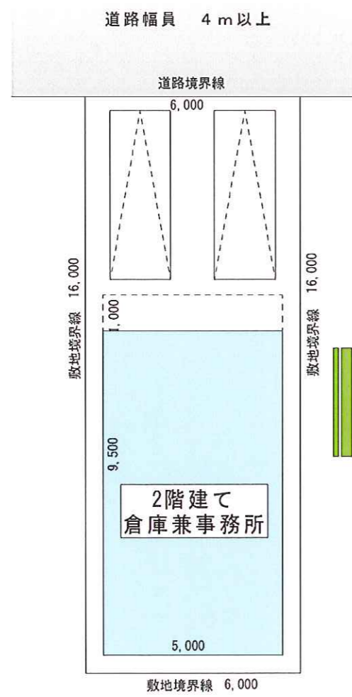
平面配置図
