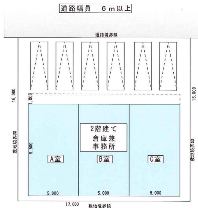
平面配置図
